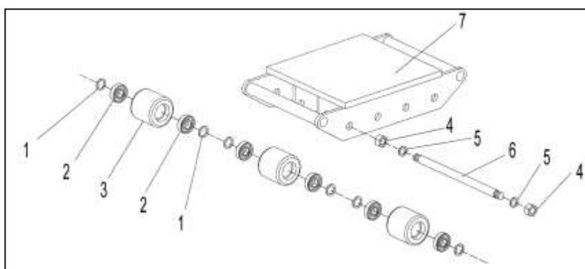
Схема 6. Платформа такелажная CRO-12
